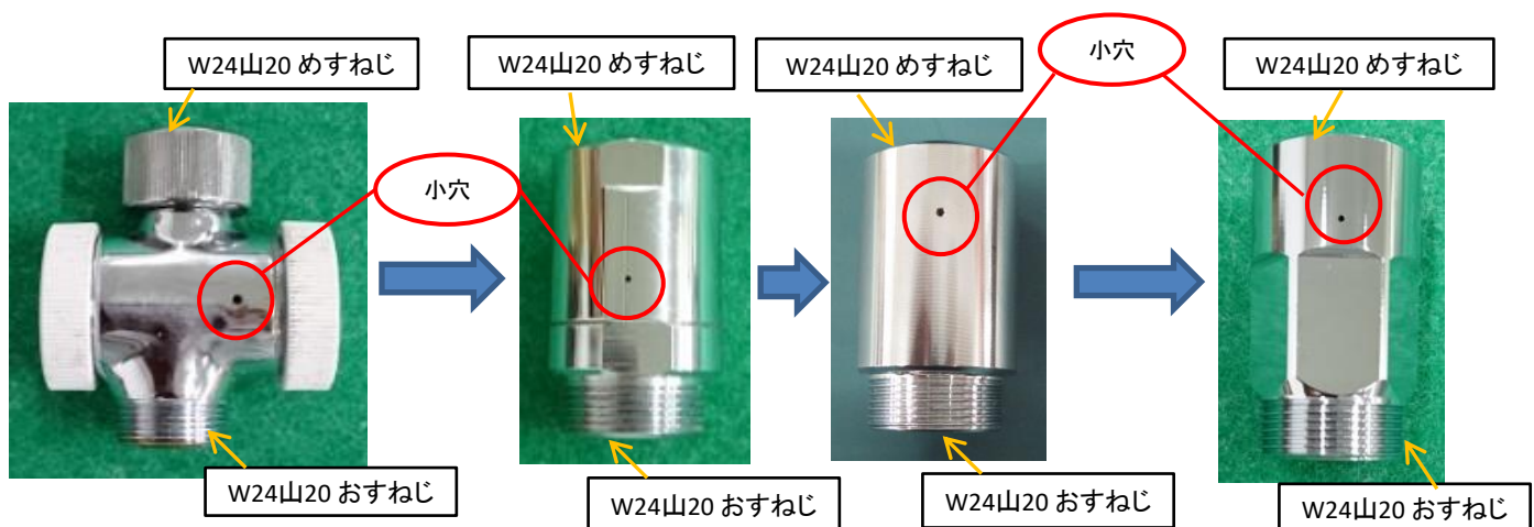
現行品の調圧弁
