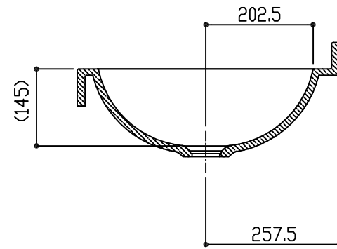
A-A 断面
