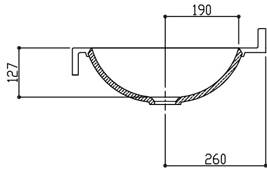
A-A 断面
