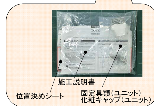
サイドカバーユニット
