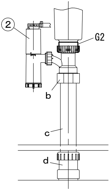
排水配管部材（参考）
