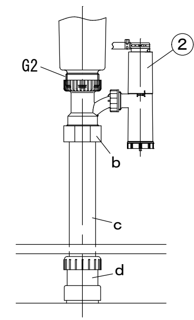
排水トラップねじ径がG2の場合
