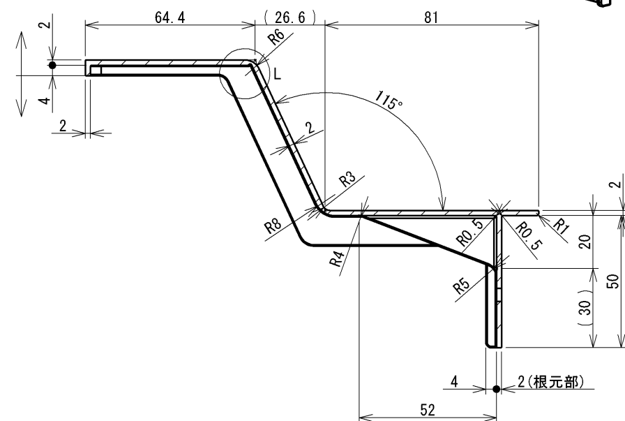
断面図 J-J
