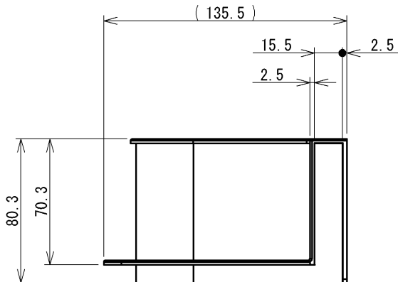
断面図 A-A
