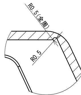
詳細図 L スケール 2 : 1
